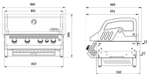
Datenblatt „Maße“ Gasgrill SANTOS Free S-410
